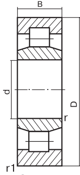
Эскиз 1 Drawing 1
