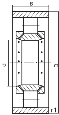
Эскиз 12 Drawing 12
