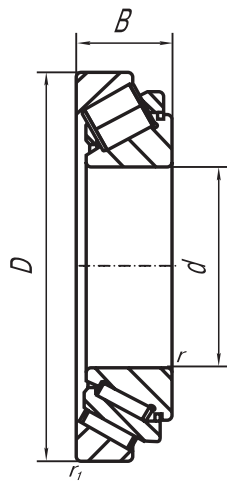
Эскиз 1 Drawing 1
