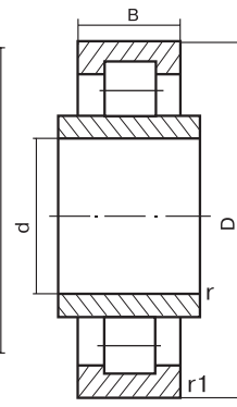
Эскиз 10 Drawing 10
