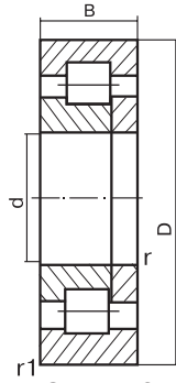
Эскиз 3 Drawing 3
