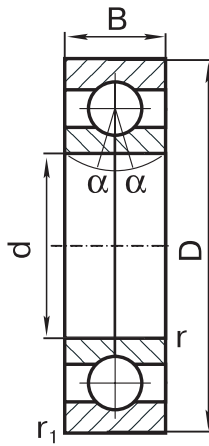
Эскиз 2 Drawing 2
