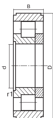
Эскиз 16 Drawing 16
