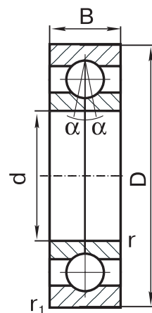
Эскиз 4 Drawing 4
