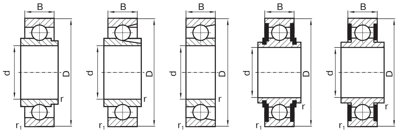
Эскиз 7 Drawing 7 Эскиз 8 Drawing 8 Эскиз 9 Drawing 9 Эскиз 10 Drawing 10 Эскиз 11 Drawing 11
