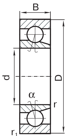
Эскиз 2 Drawing 2
