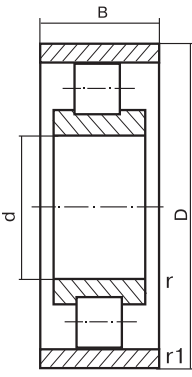
Эскиз 17 Drawing 17
