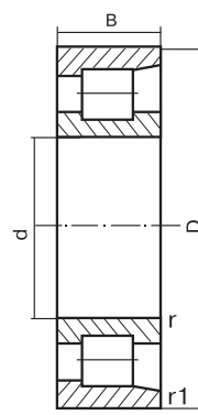
Эскиз 19 Drawing 19
