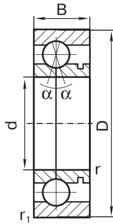
Эскиз 3 Drawing 3
